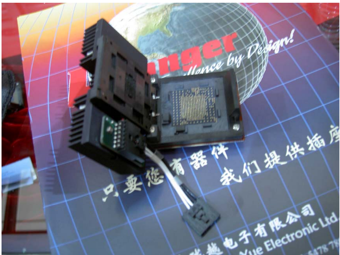
展台上展示的 SmartSocket™ 实例
