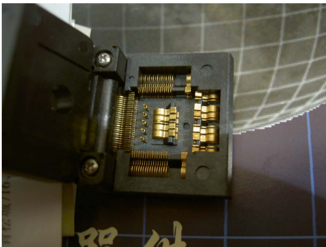
展台上展示的混合技术构成的测试/老化插座实例
