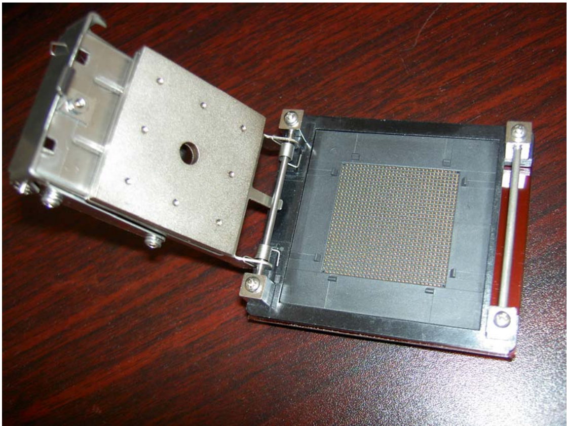
展会上展示的 1020 球的 BGA 插座
