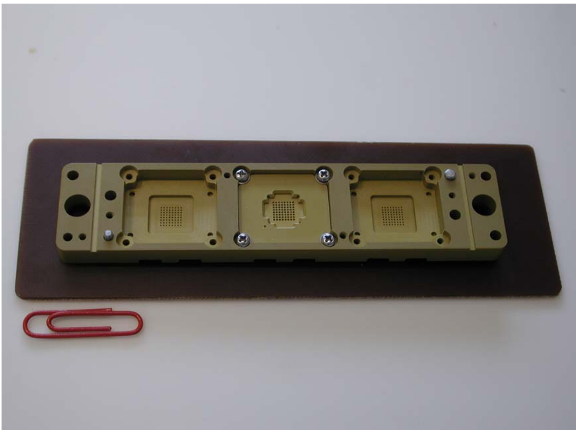
用于自动测试的三种不同封装类型的并行测试连接器
